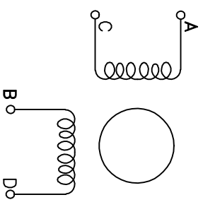
绕组接线示意图
